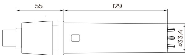
VERTEX-R™ VC-R4
